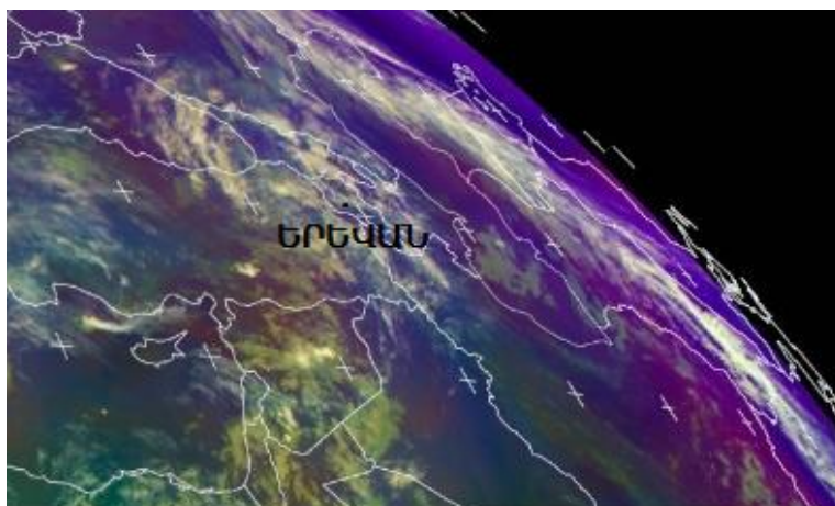
Երկրի արհեստական արբանյակից ստացված ամպամածության պատկերը (23.10.2018թ. ժ.10.00)
